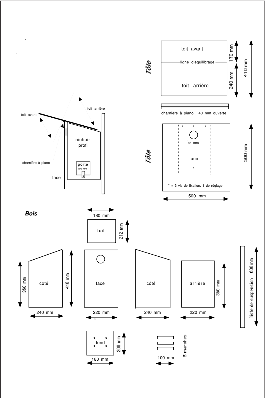
Plan du nidhoir à toit basculant.
